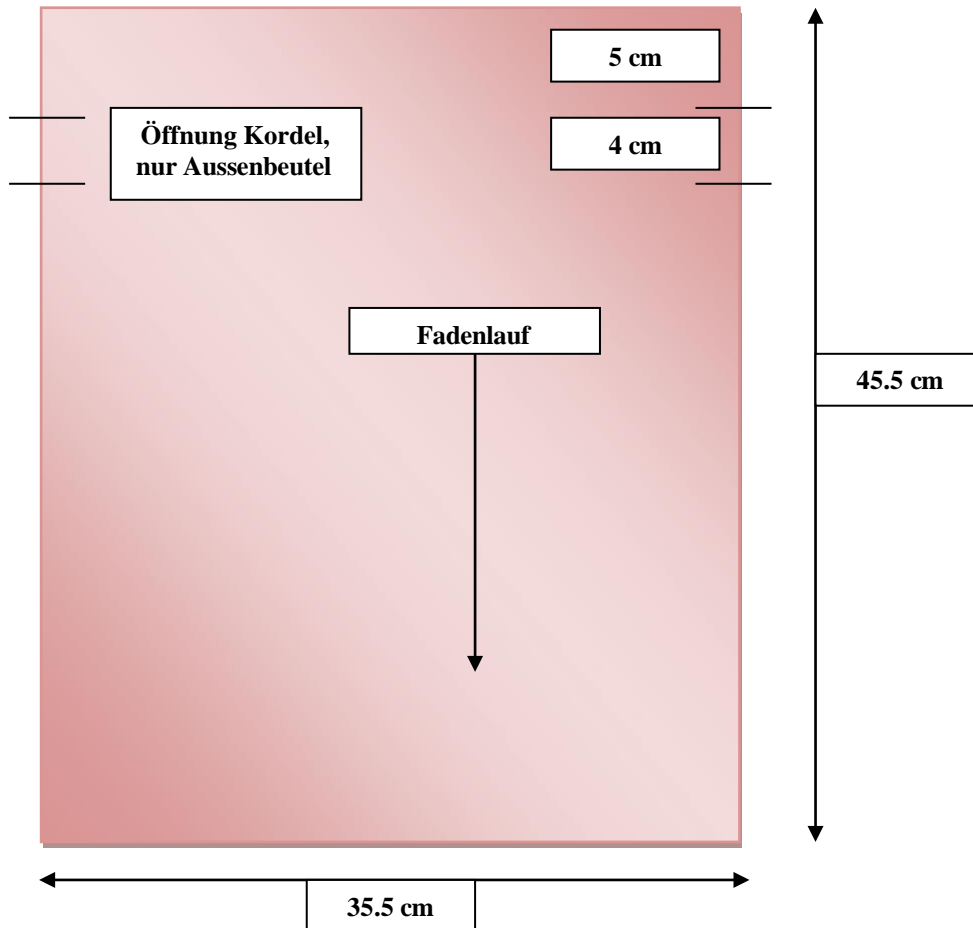
Schnittteil 2
